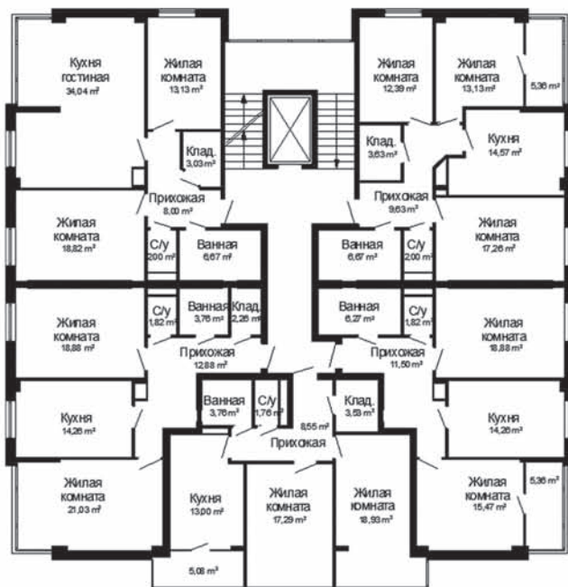
Варианты планировок
